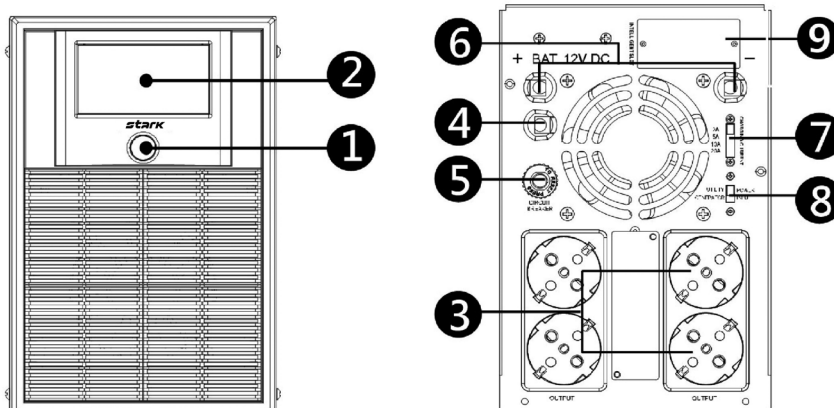
Вид спереди
